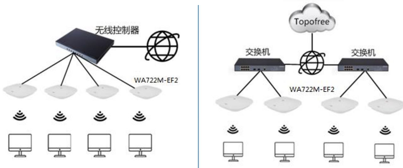
集中管理（本地AC与敦崇云平台）
